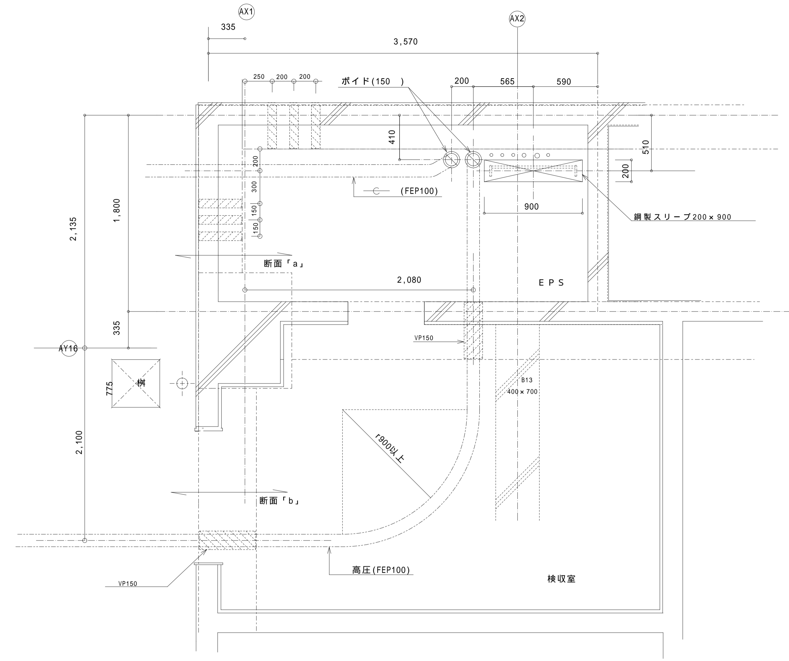
EPS高圧地中配管・2 F 床開口図 1/20
