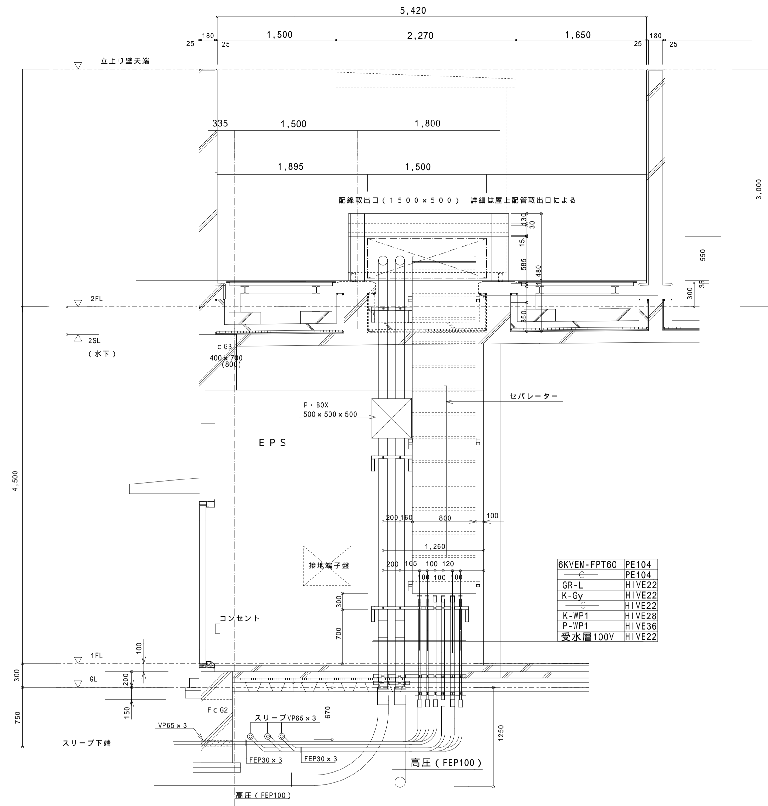
E P S 断面「a」図 1/30
