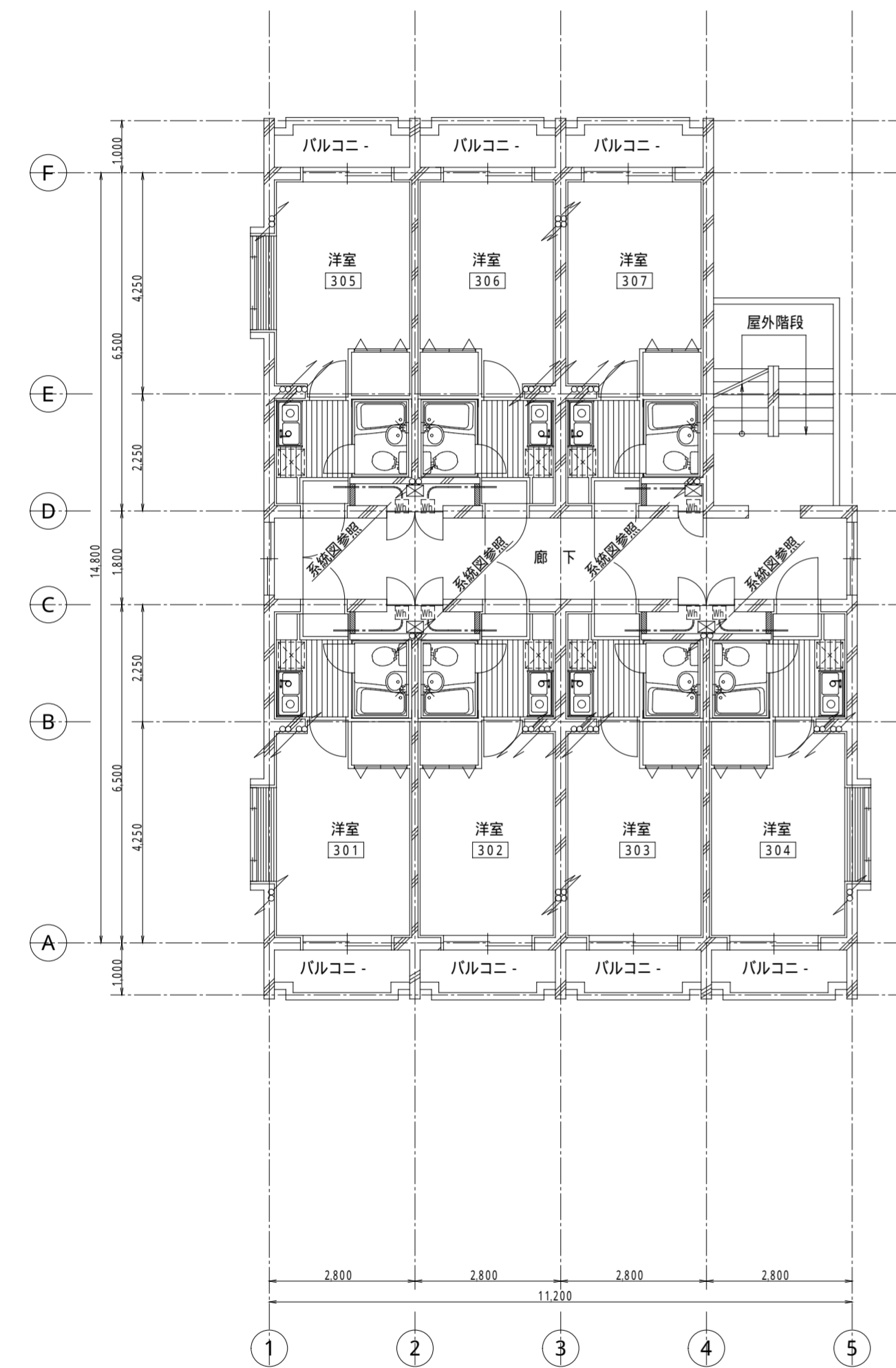
3階 平面図
