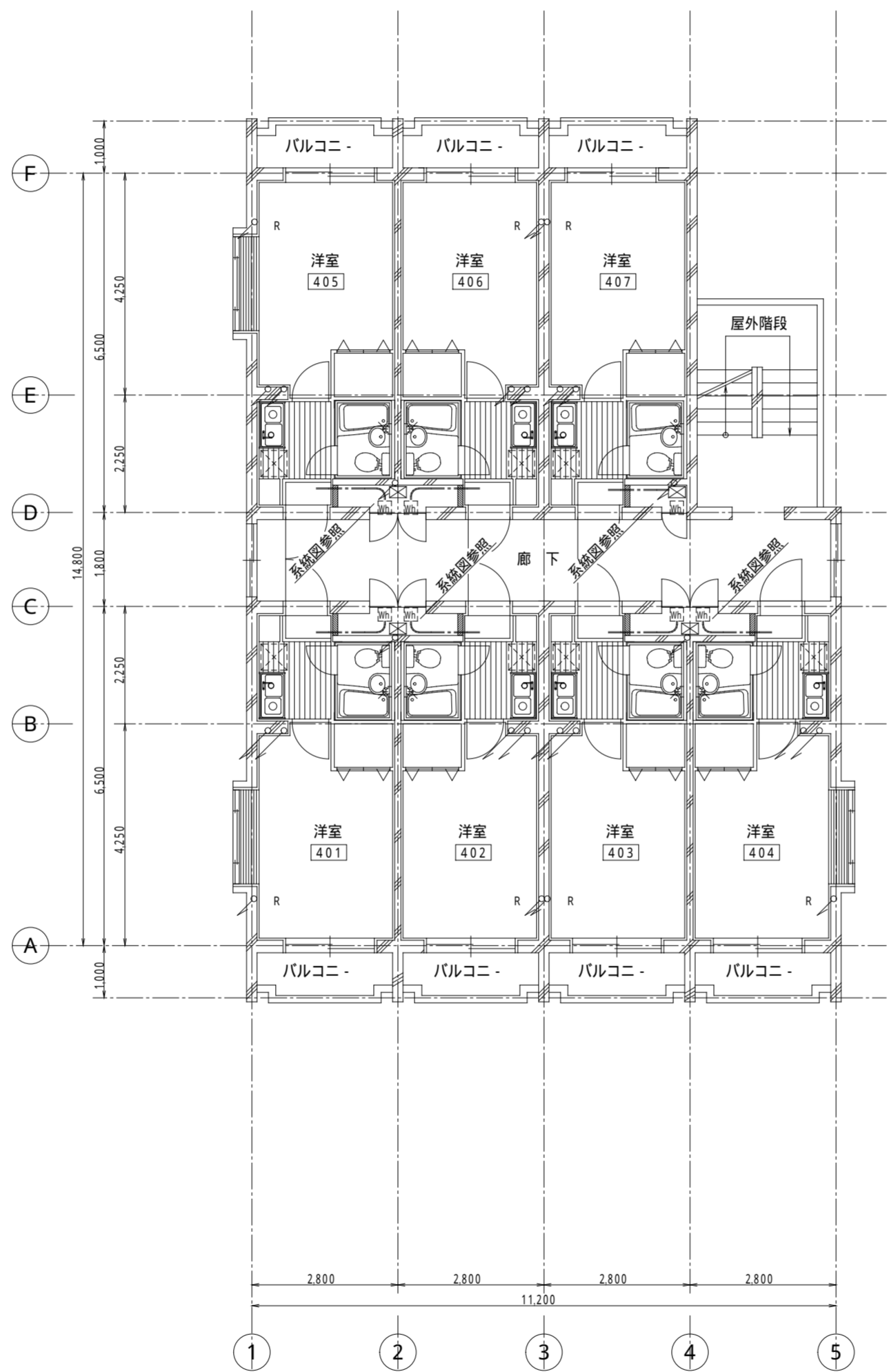
4階 平面図
