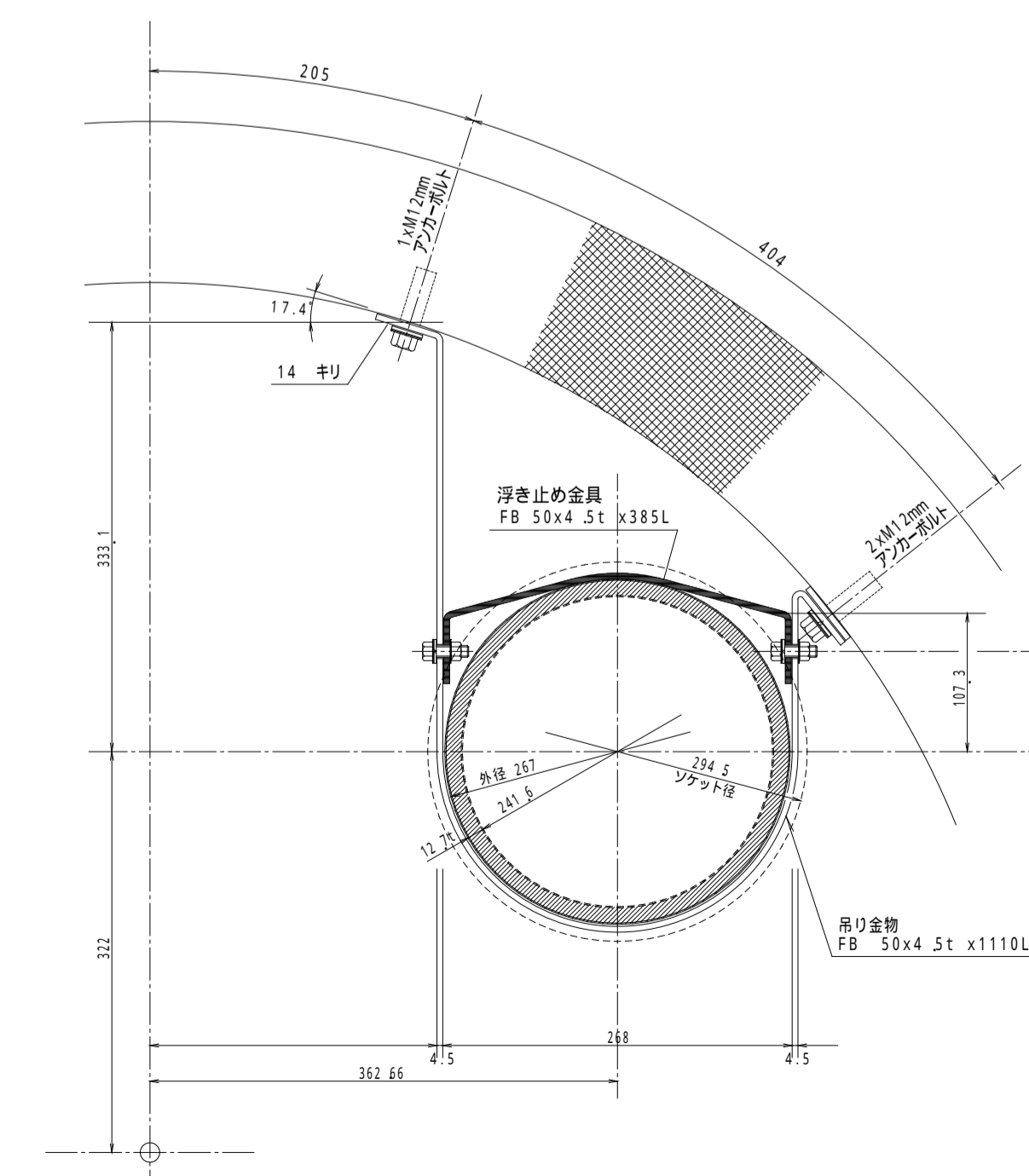
部分詳細図 S=1/5
