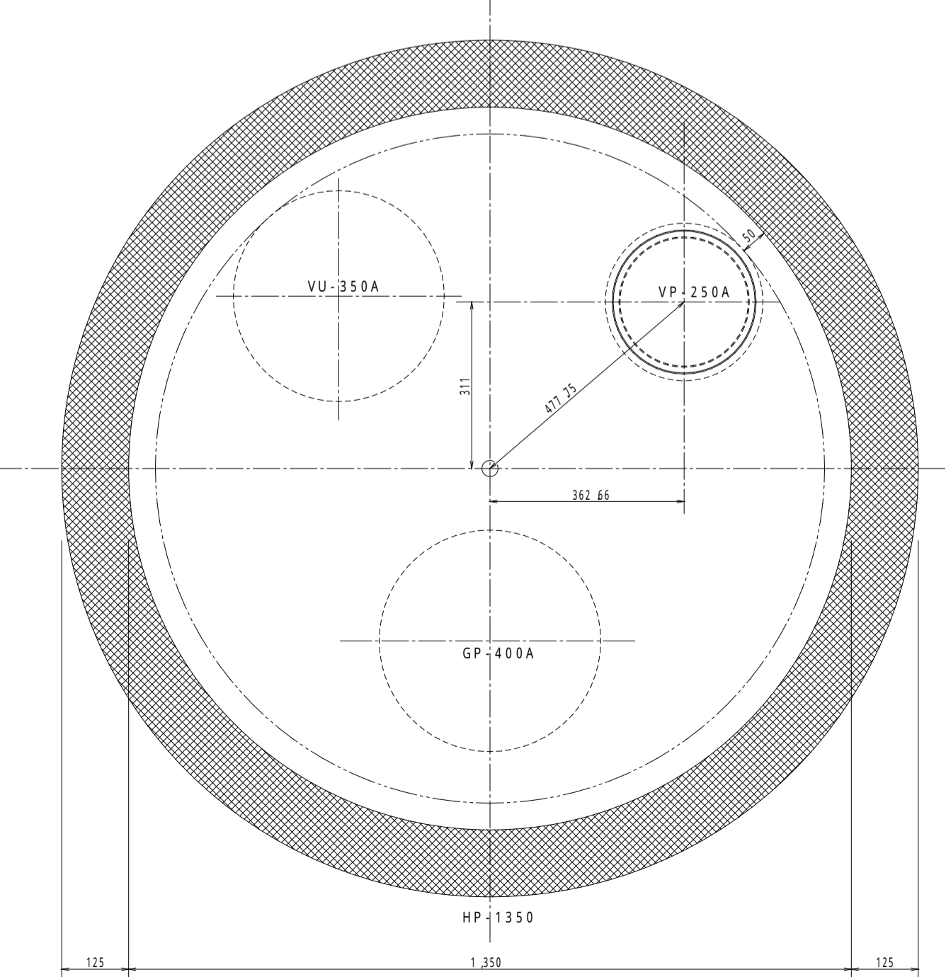
断面詳細図 S=1/10
