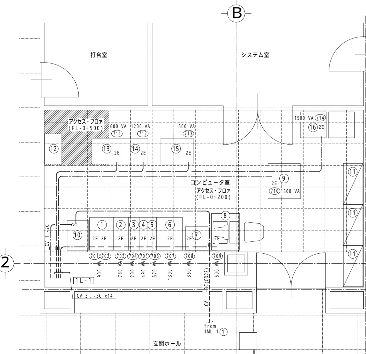
3 コンピュータ室 配線図 (コンセント設備) 1/50
