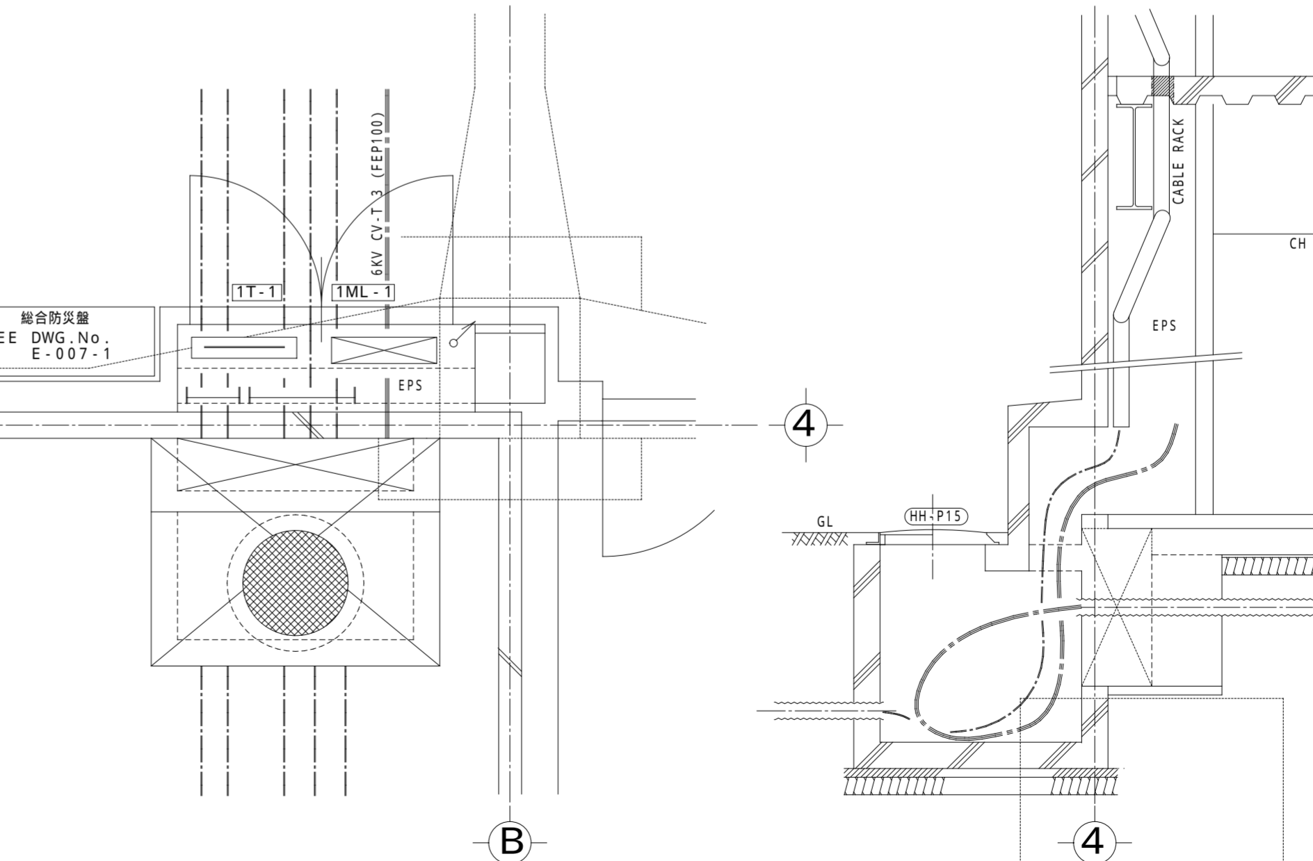
4 引込ハンドホール詳細図 (HH-P15) 1/30
