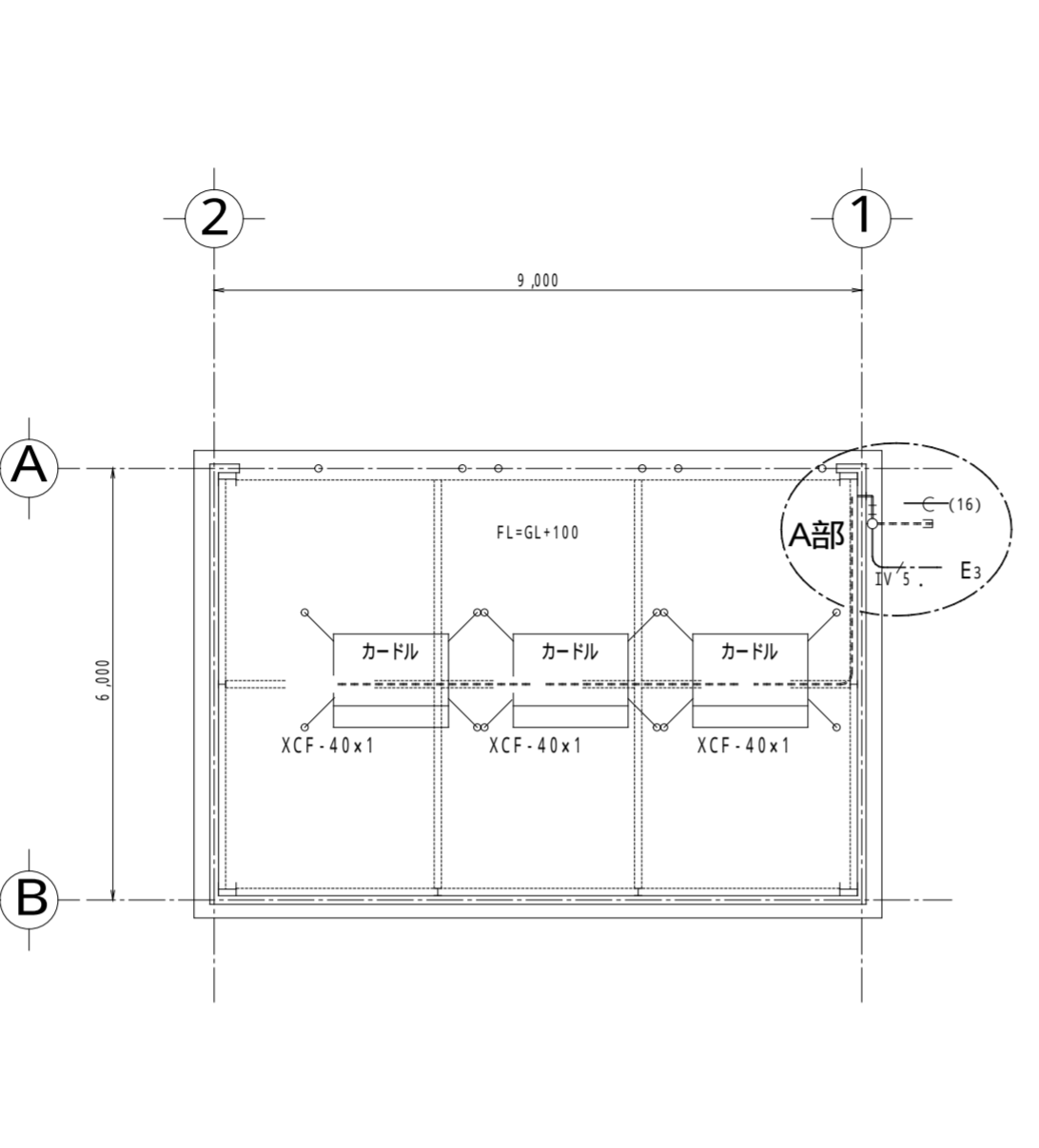
2 高圧ガス(水素)貯蔵庫配線図 (照明設備) 1/100
