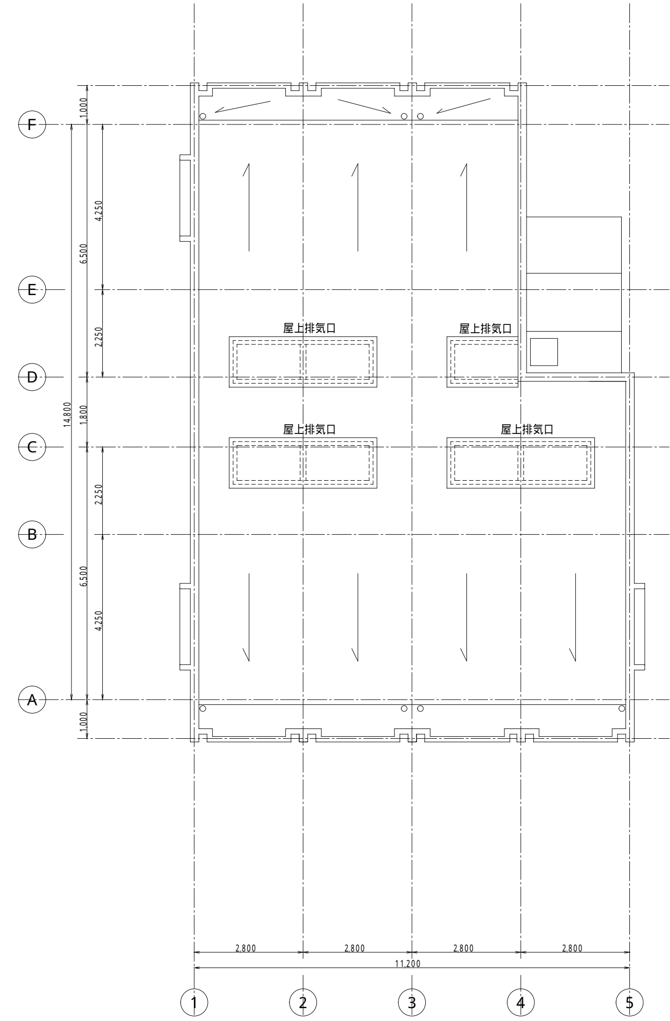
R階 平面図
