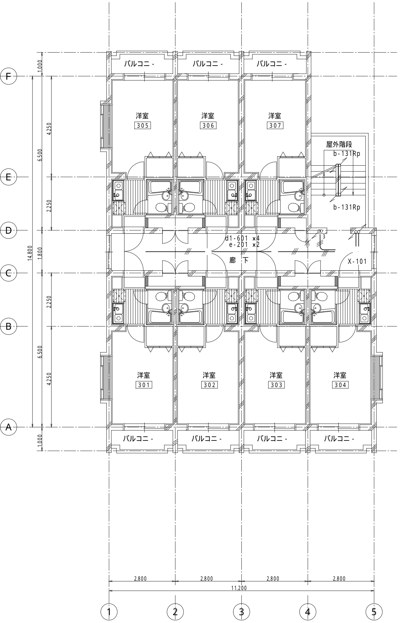
3階 平面図
