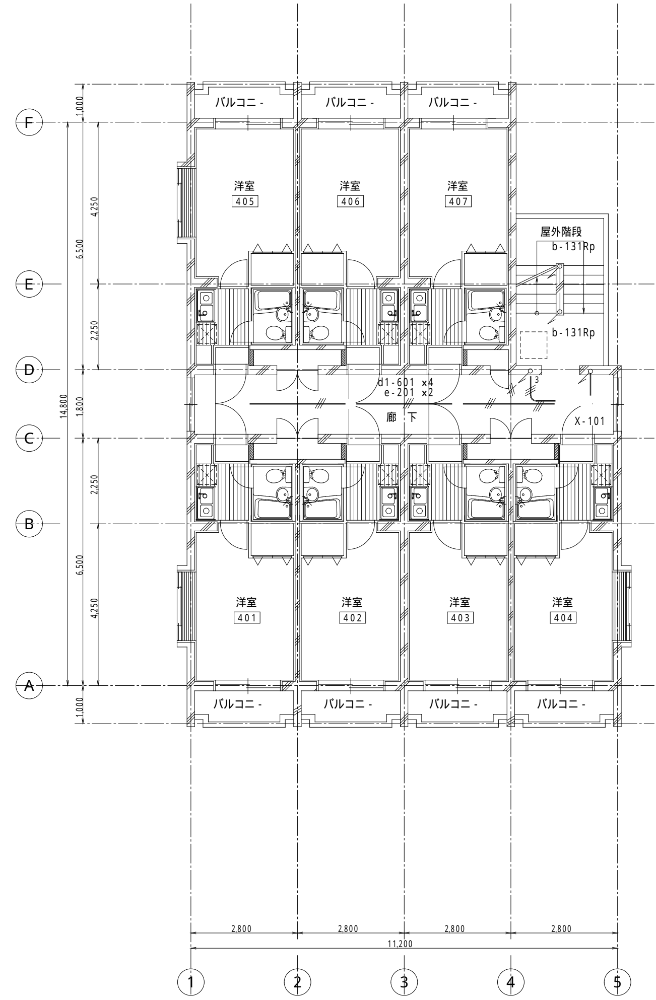
4階 平面図
