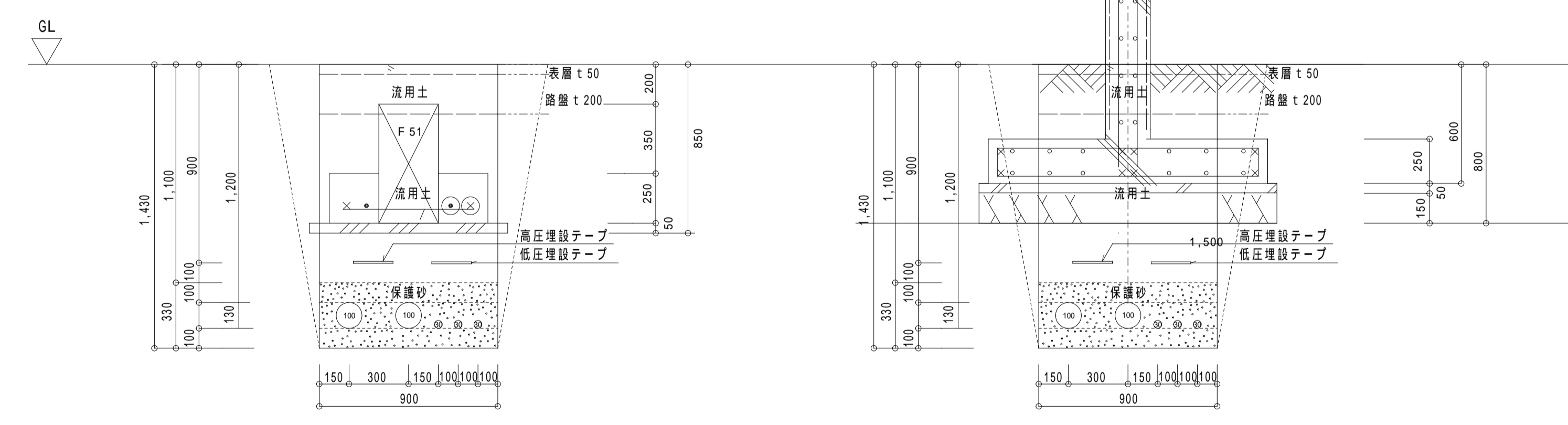
地中配管 a
