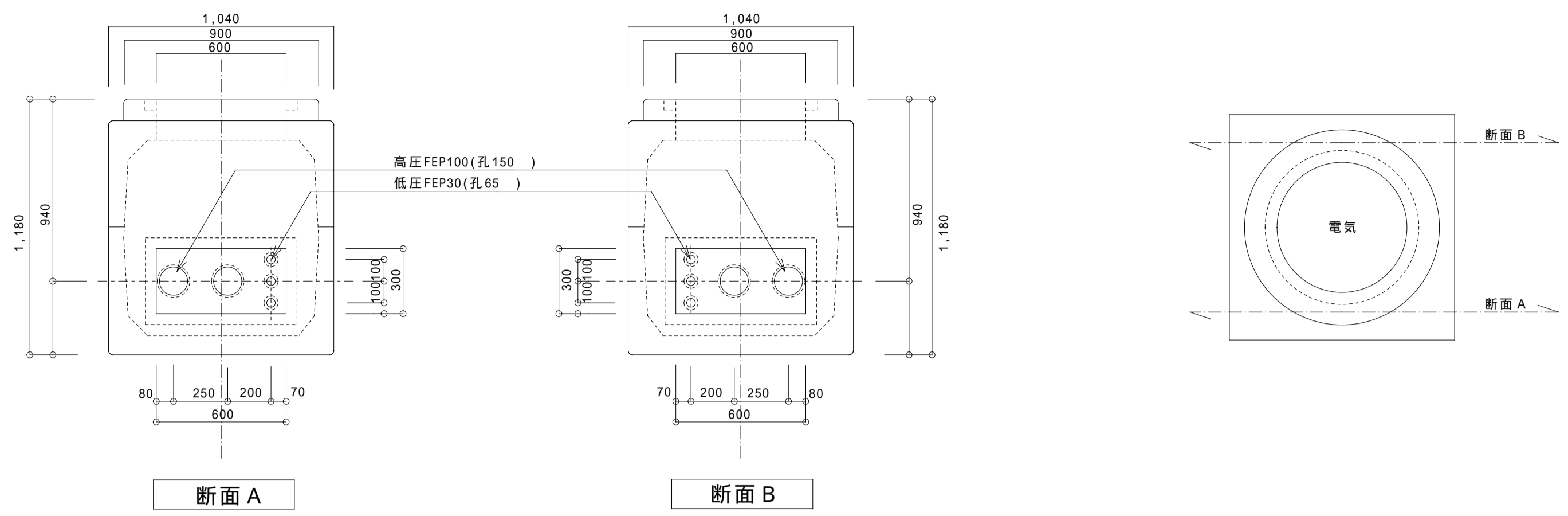
ハンドホール「B」孔アケ加工図
