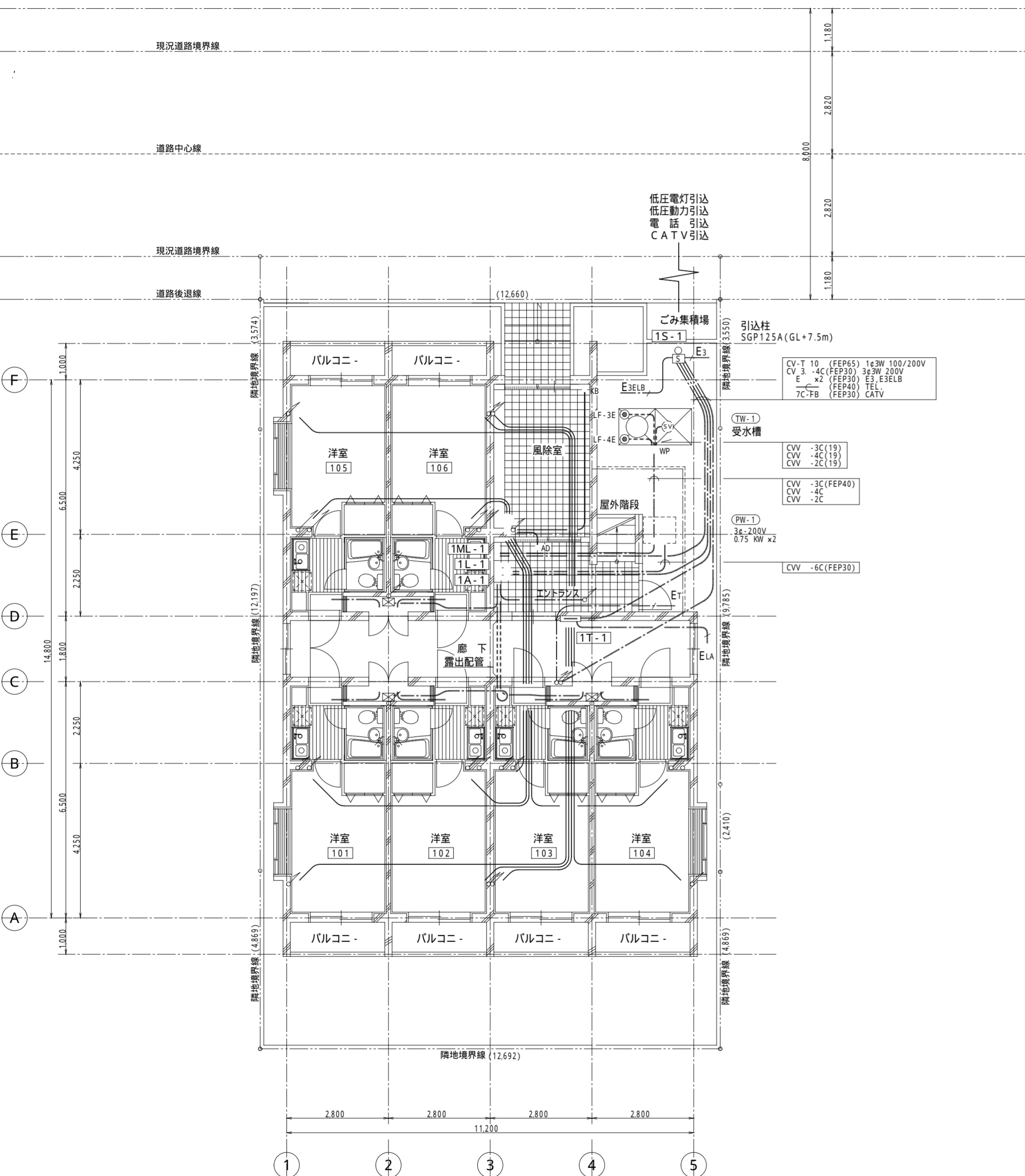
1階 平面図
