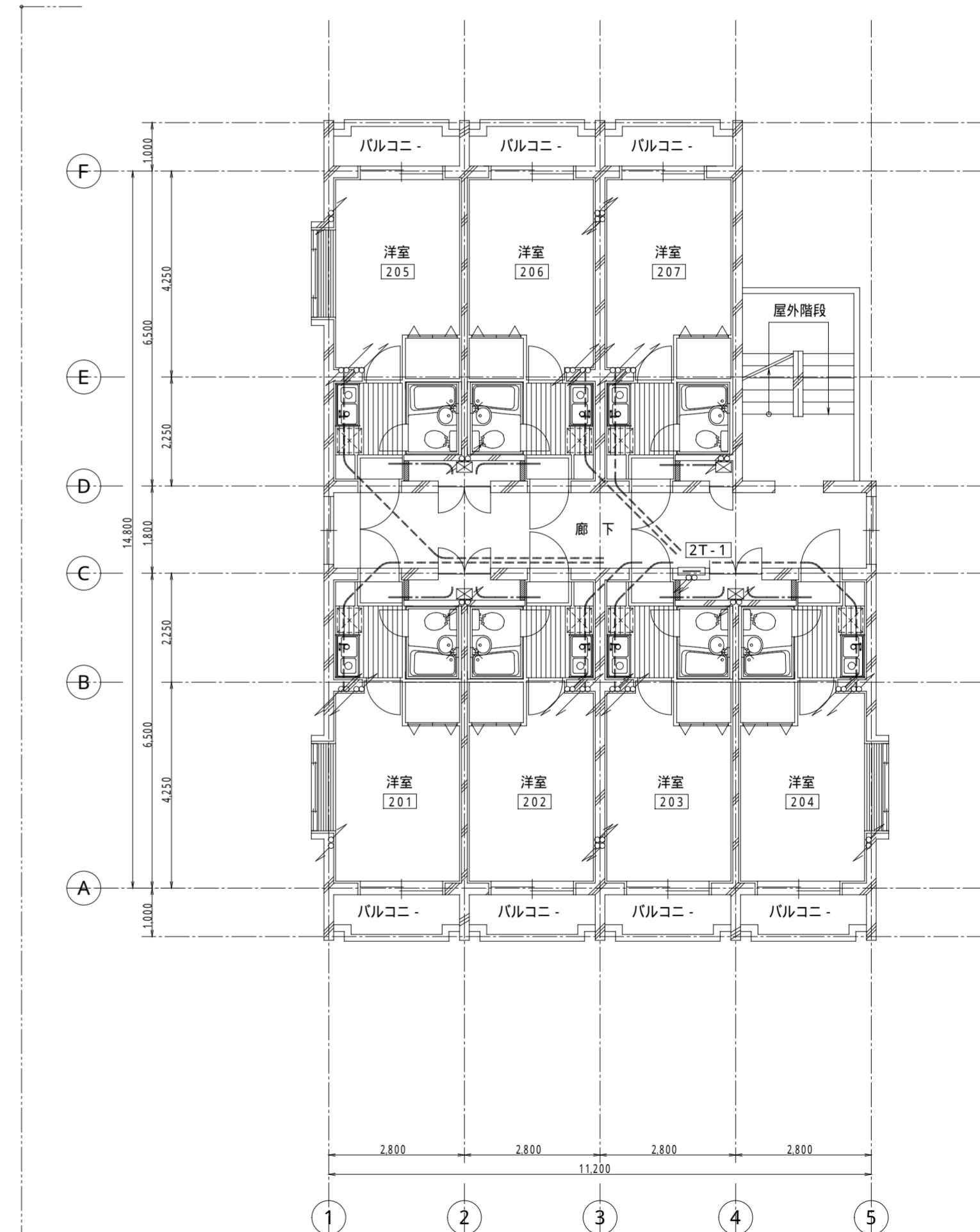
2階 平面図
